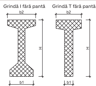
SECȚIUNI GRINZI FĂRĂ PANTĂ
