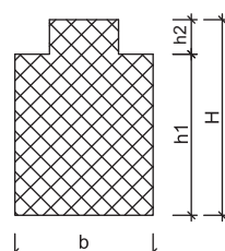
SECȚIUNE GRINDĂ PLANȘEU TIP "T"
