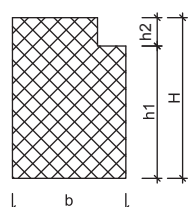
SECȚIUNE GRINDĂ PLANȘEU TIP "L"
