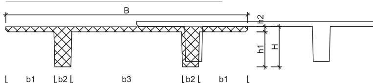
SECȚIUNE ELEMENT DE PLANȘEU TIP "TT"
