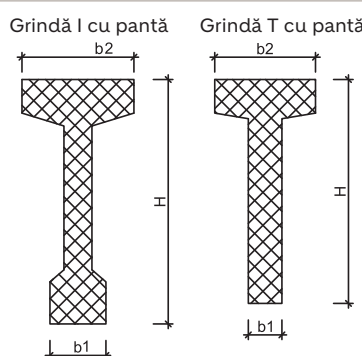
SECȚIUNI GRINZI CU PANTĂ
