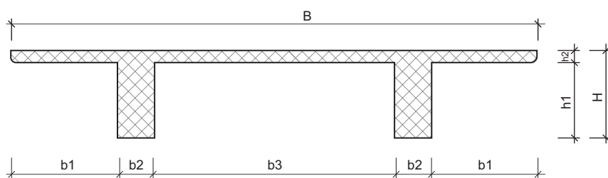
SECȚIUNE ELEMENT DE PLANȘEU TIP TT
