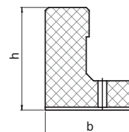
SECȚIUNE TRANSVERSALĂ C-C
