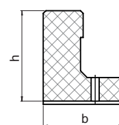
SECȚIUNE TRANSVERSALĂ A-A
