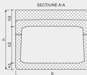
SECȚIUNE A-A
