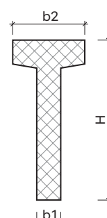
Grindă T fără pantă
