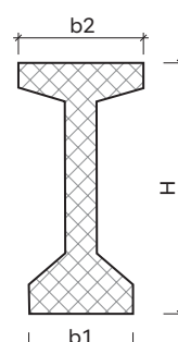
Grindă I fără pantă
